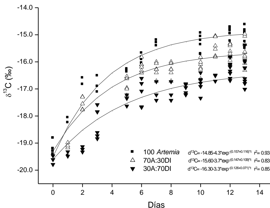
Fig. 6. Cambios en los valores isotópicos ( \delta^{13}C ) de S. senegalensis después de un cambio dietario (10 DPE) de rotíferos a Artemia y dos regímenes de co-alimentación incluyendo Artemia y alimento inerte. Valores predichos por el modelo de Hesslein fueron ajustados a valores observados usando regresión no-lineal iterativa. (Gamboa-Delgado et al. 2008).
